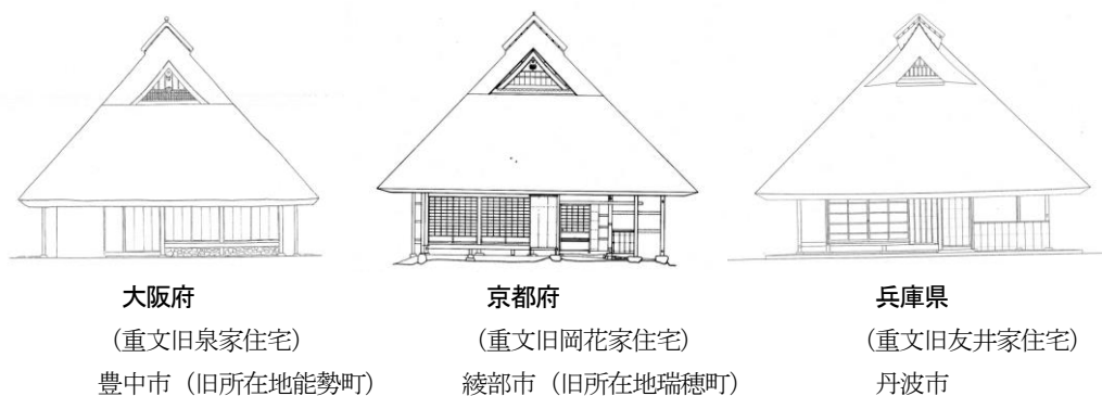
図4 各地の撰丹型民家の屋根と破風の大きさ
